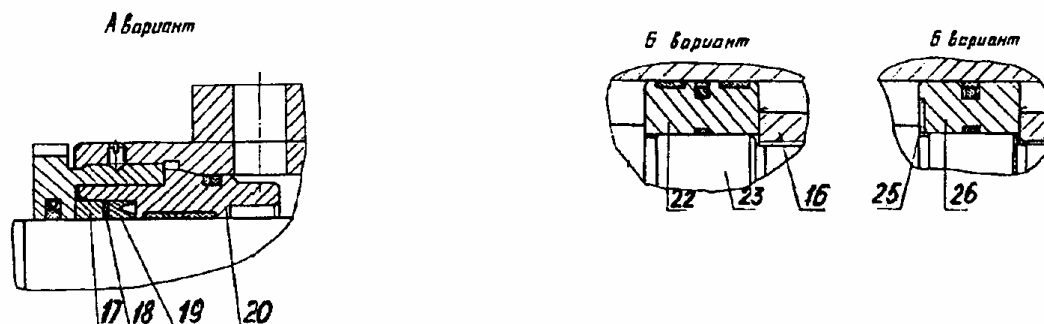
Рис. 35 Гидроцилиндр
