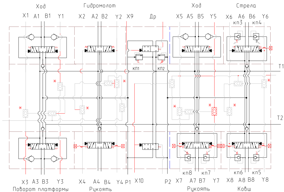
Рис. 27 Схема гидравлическая гидрораспределителя P - подвод, А и В - отводы, X и Y – линии управления, Т – слив, Др – дренаж.
