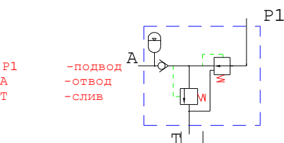
Рис. 37 Пневмогидроаккумулятор
