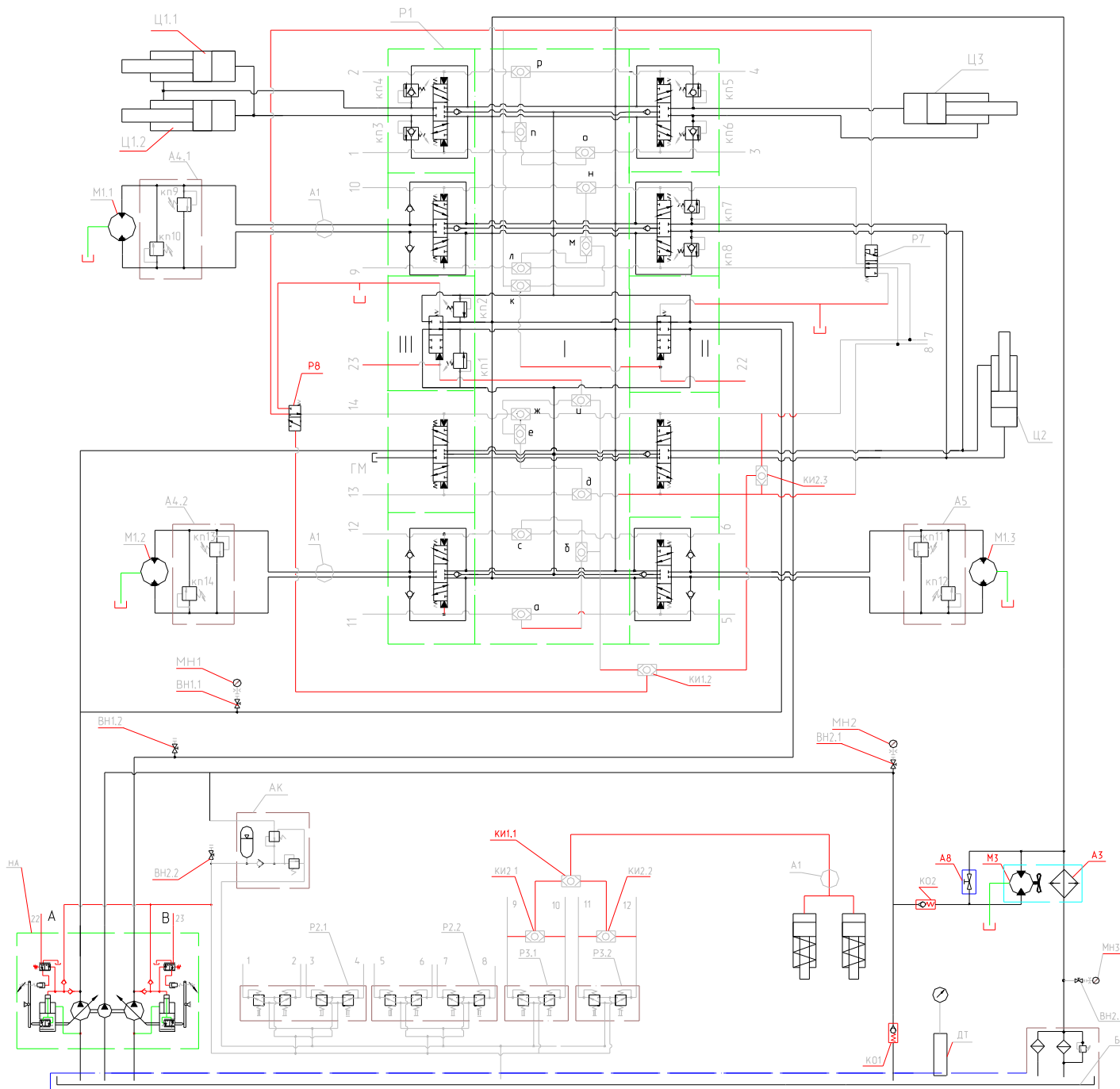
Рис. 22 Принципиальная гидравлическая схема
