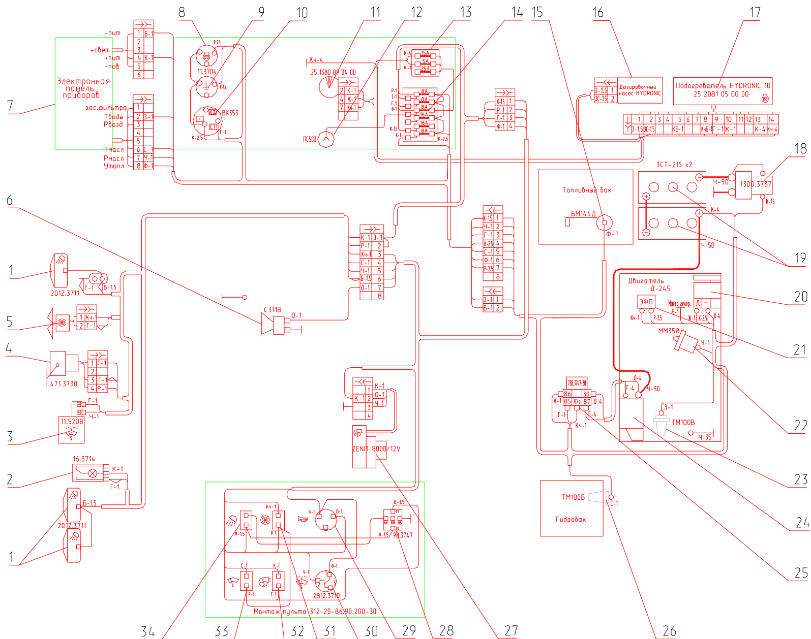
Рис. 44 Электрическая схема экскаватора
