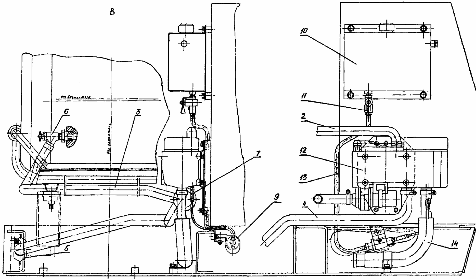
Рис. 26.2 Установка предпускового подогрева двигателя и отопления кабины
