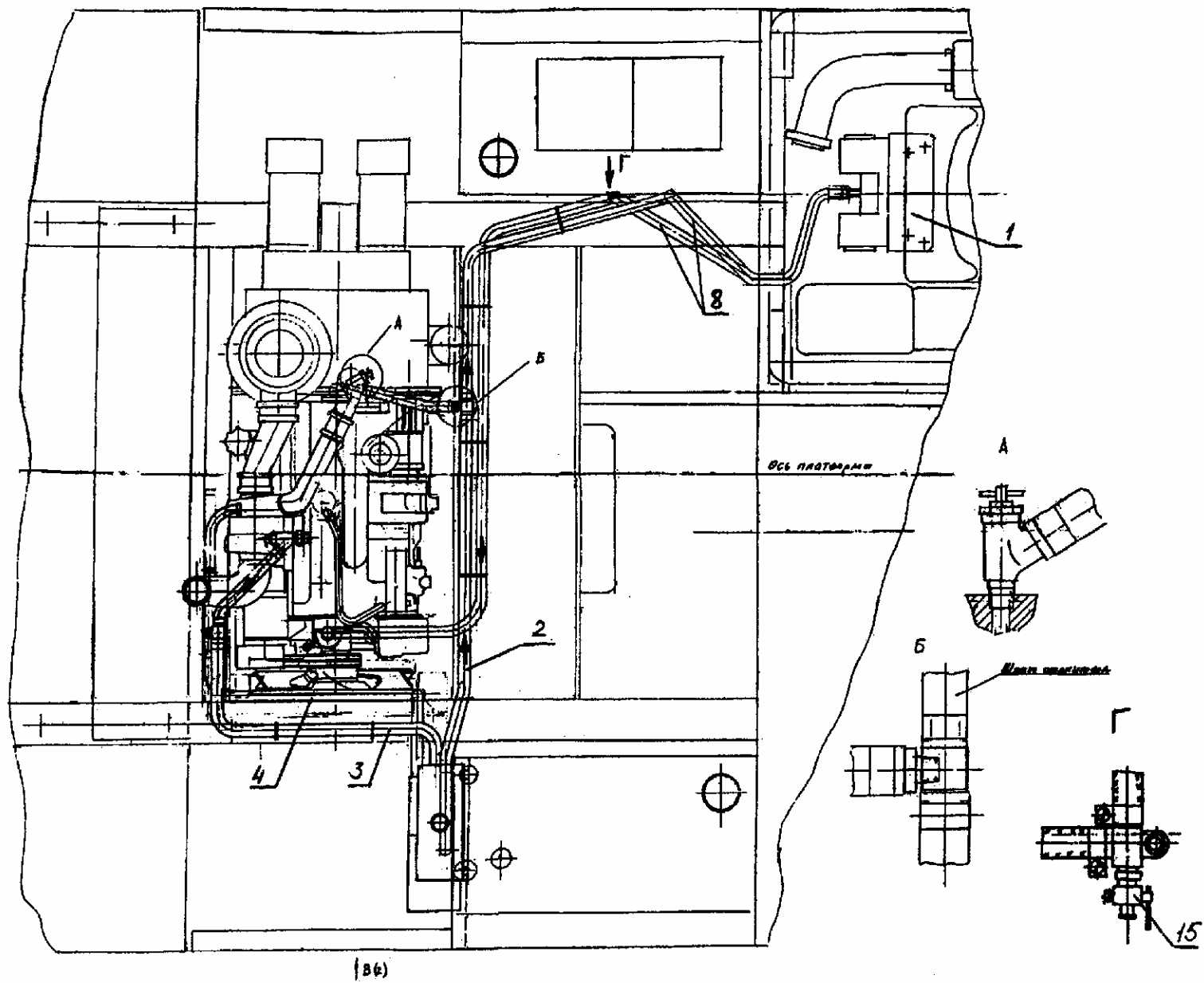
Рис. 26.1 Установка предпускового подогрева двигателя и отопления кабины
