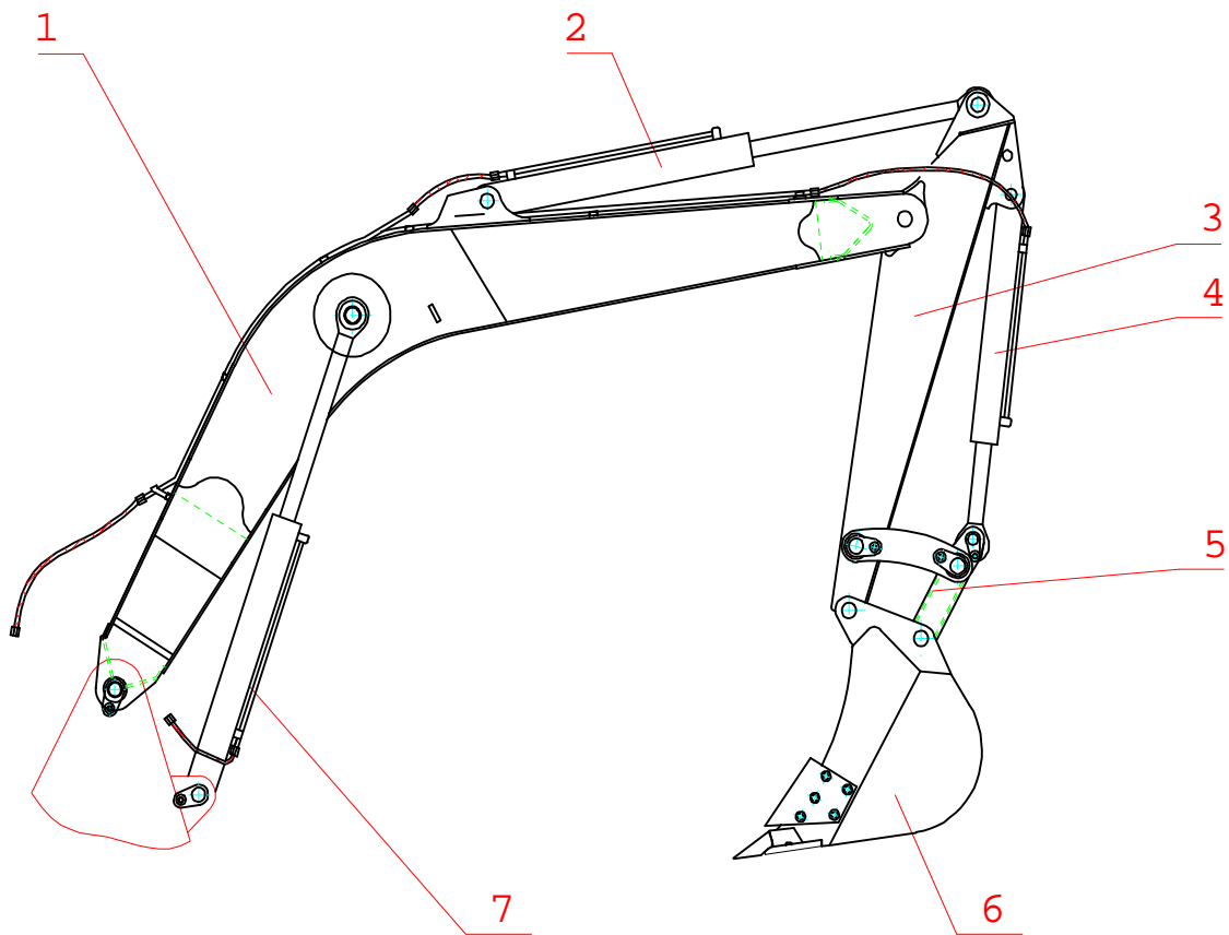
Рис. 21 Рабочее оборудование обратная лопата 1 - стрела; 2, 4, 7 - гидроцилиндры; 3 - рукоять; 5 - механизм привода ковша; 6 - ковш
