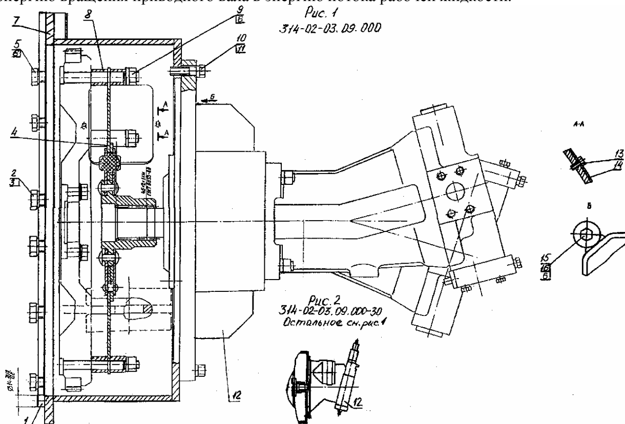
Рис. 23 Установка насоса
