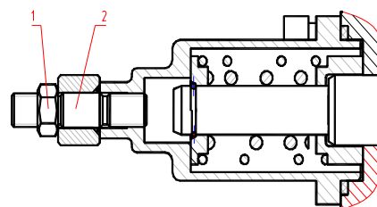
Рис. 9 Ограничитель хода золотника гидрораспределителя 1 - гайка; 2 - шпилька.
