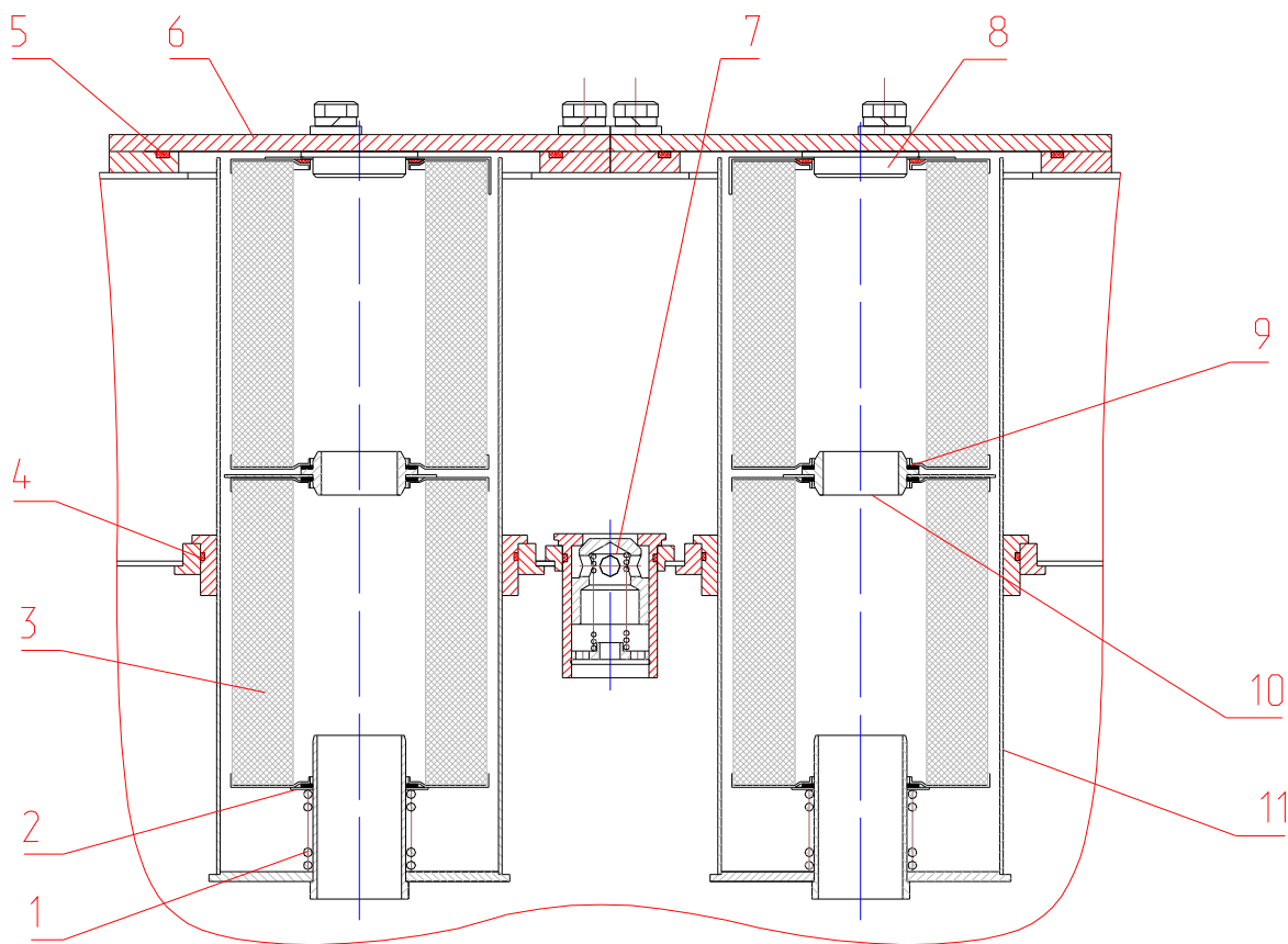
Рис. 41 Фильтр магистральный
