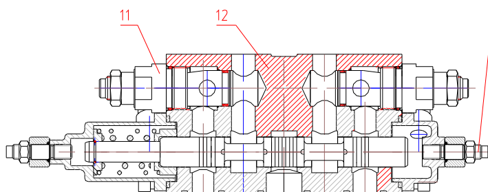
Рис. 30 Рабочие секции гидрораспределителя
