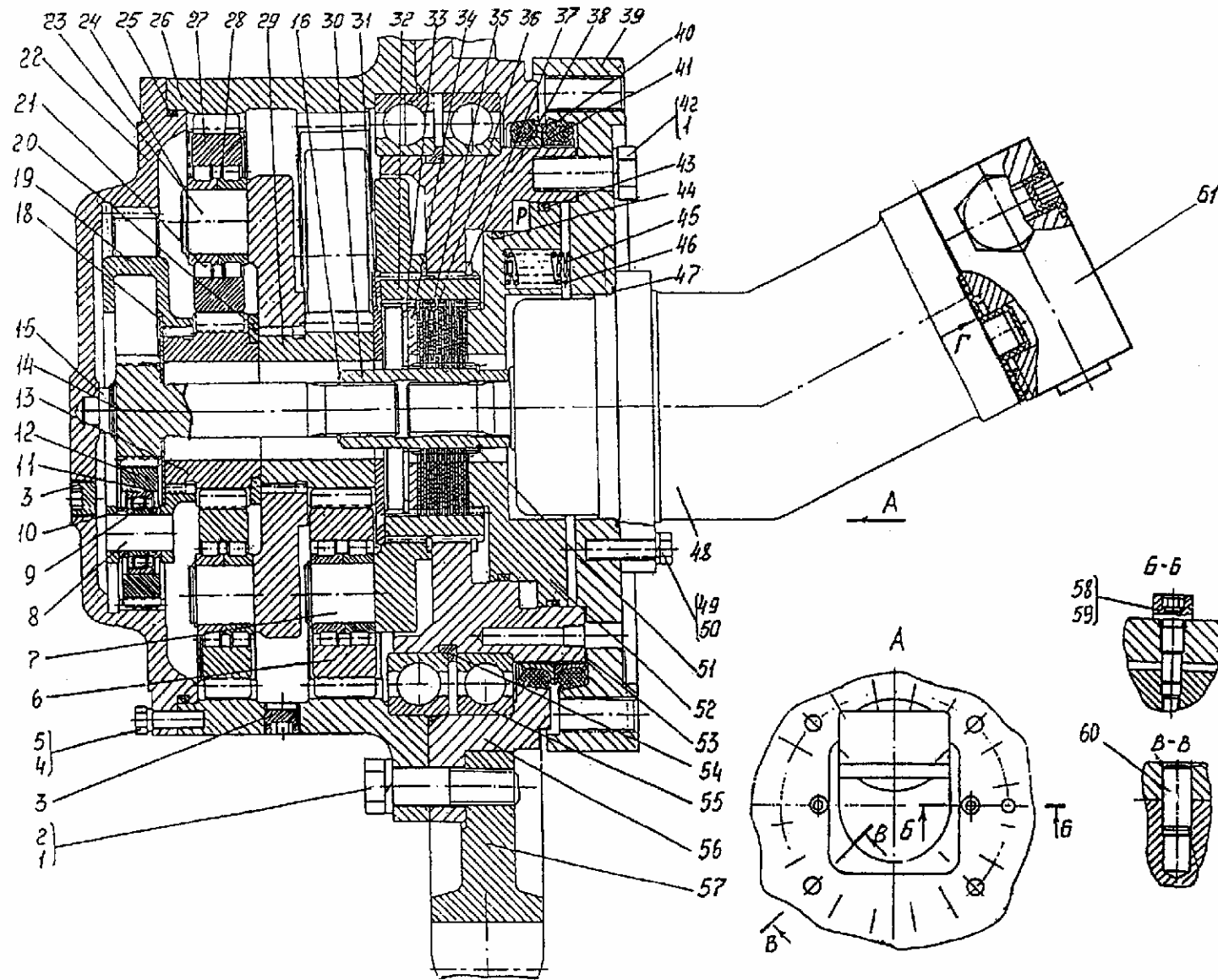
Рис. 14 Привод хода
